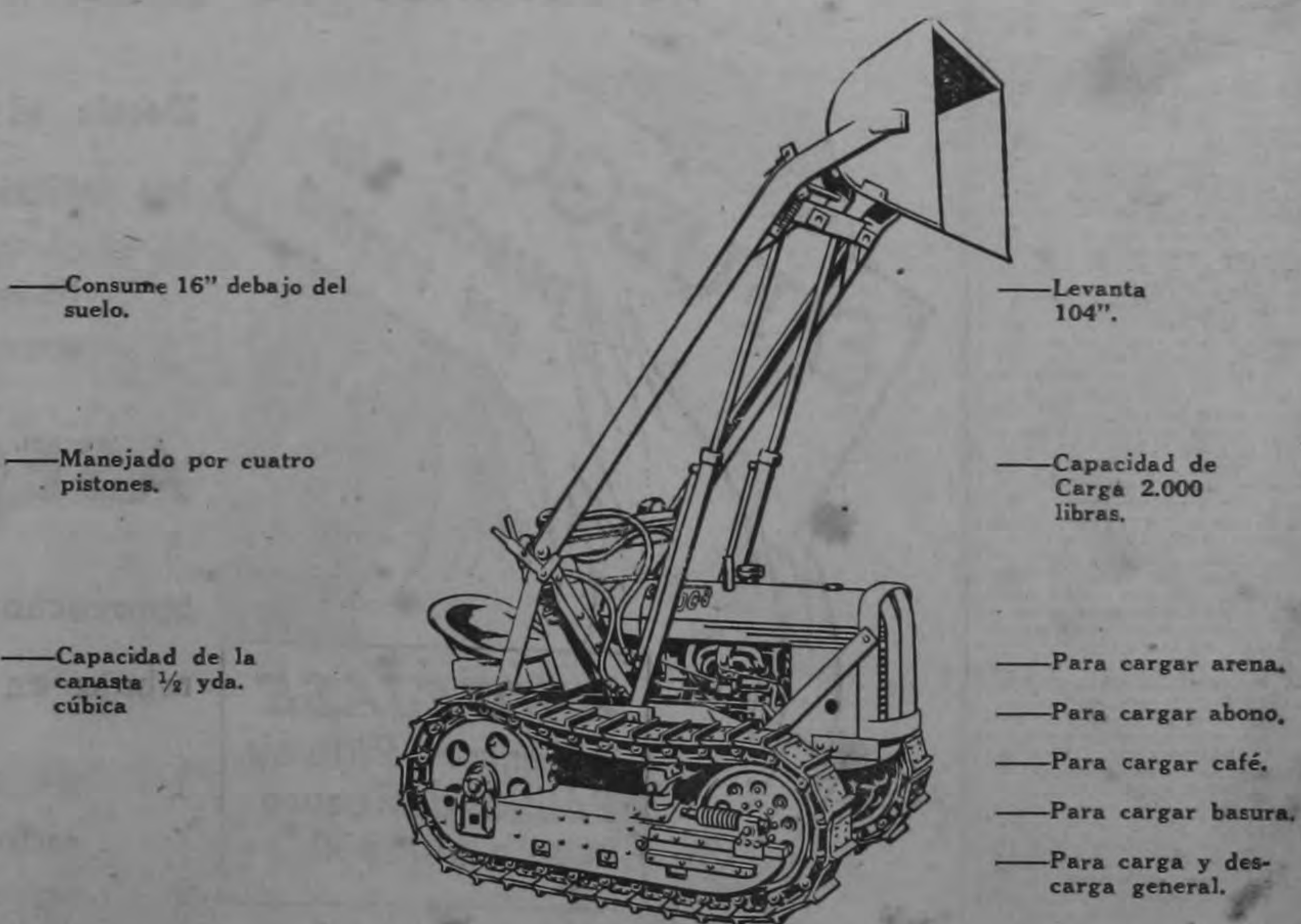
El Cargador Hidráulico "OLIVER". Montado Sobre Tractor Oliver de Oruga
